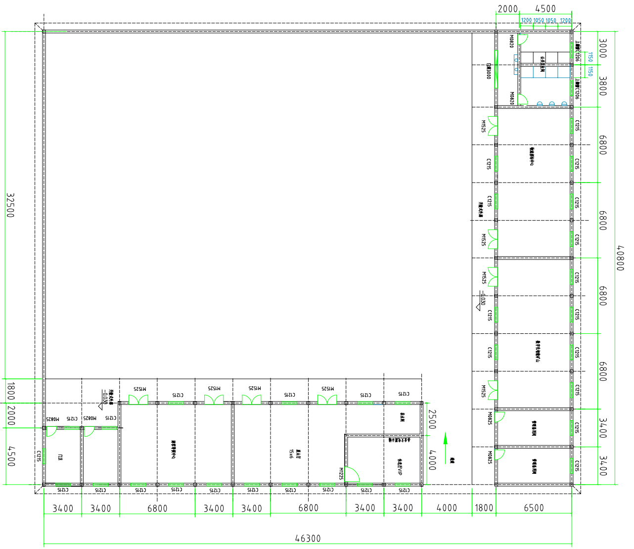
进岛广场用房平面布置图
